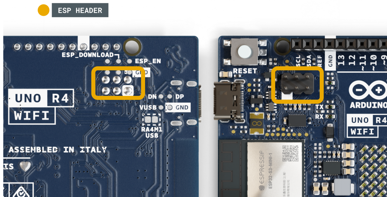
ESP header.
